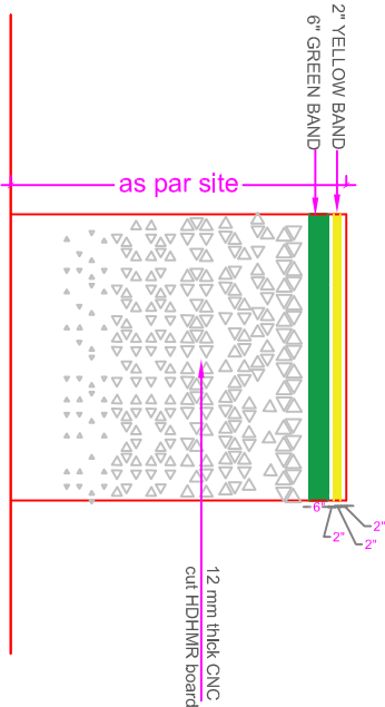
ELEVATION - A
