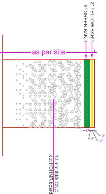
ELEVATION - D
