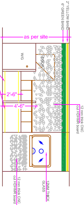
ELEVATION - A
