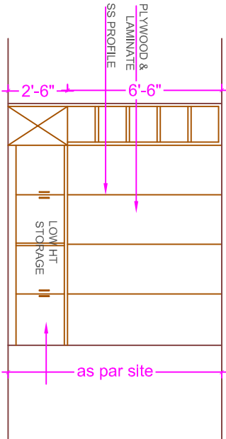
ELEVATION - B
