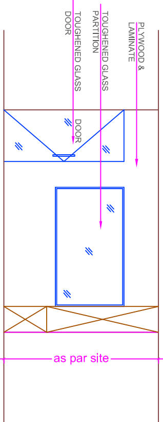
ELEVATION - D
