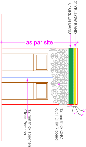
ELEVATION - C
